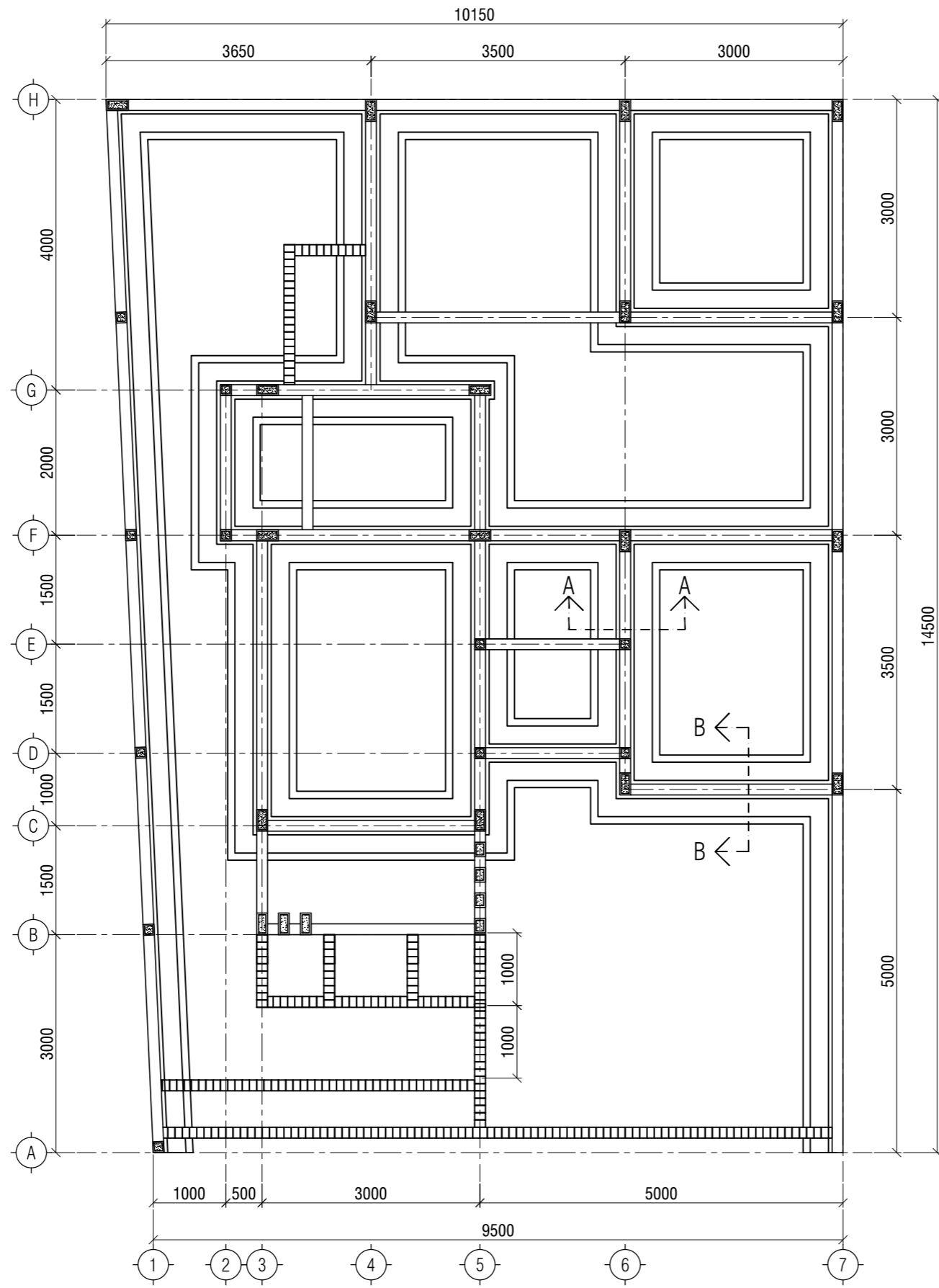
1 DENAH PONDASI SKALA 1:75
